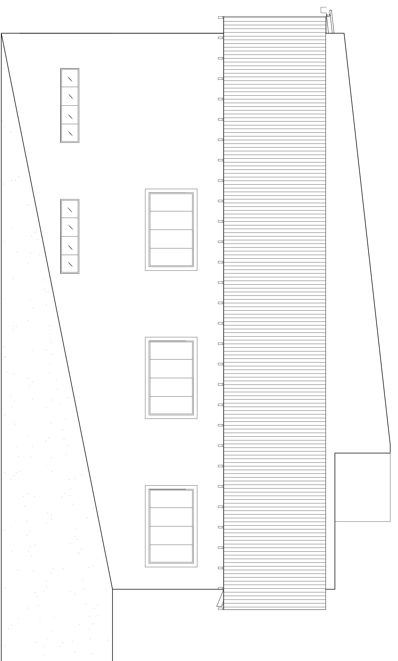
FACHADA 2 ESCALA 1:50
